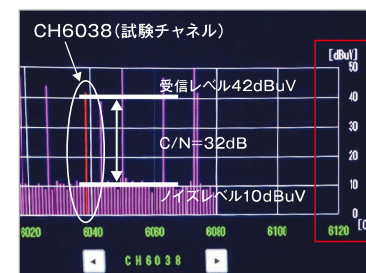
《図1》簡易スペアナ表示例
